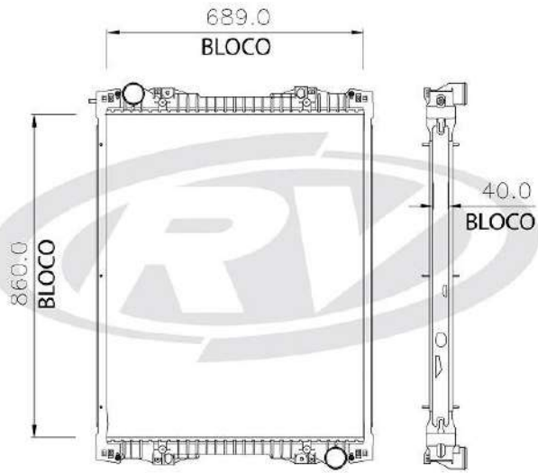
12047 SCANIA
