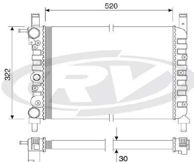
12531 FIAT
