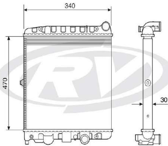
12508 VOLKSWAGEN
