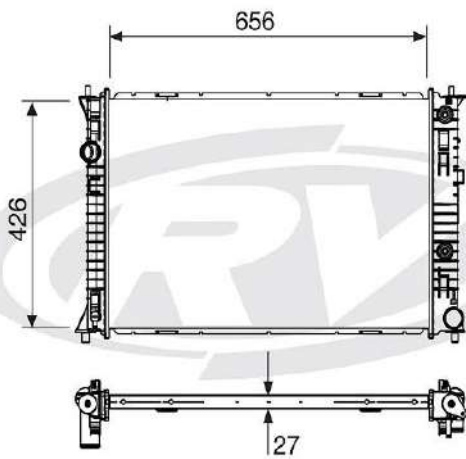
12737 FORD
