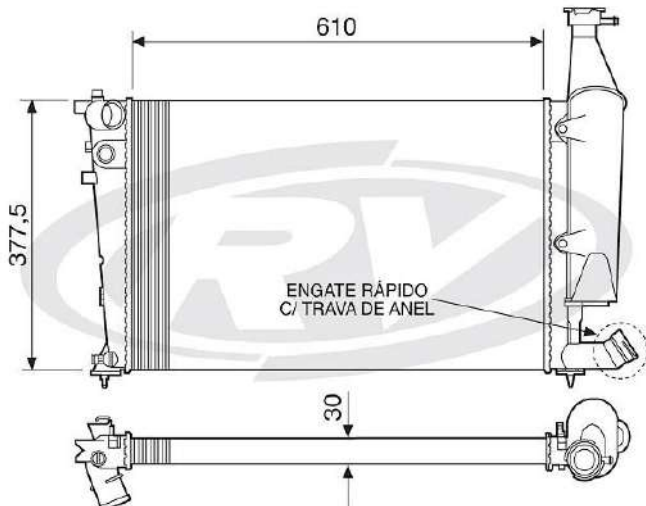
12767 CITROËN / PEUGEOT
