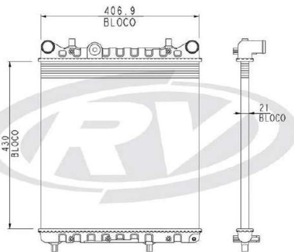
12527 VOLKSWAGEN
