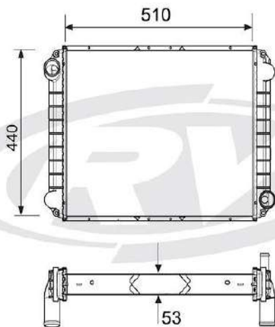
12551 IVECO
