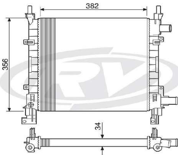
12586 FORD
