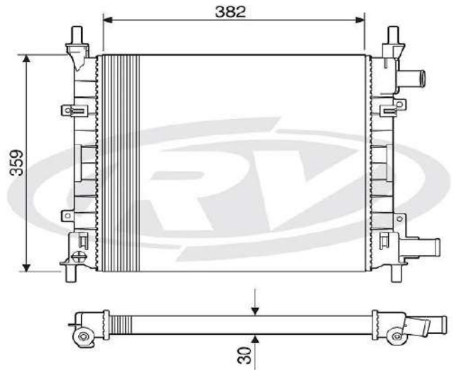
12585 FORD
