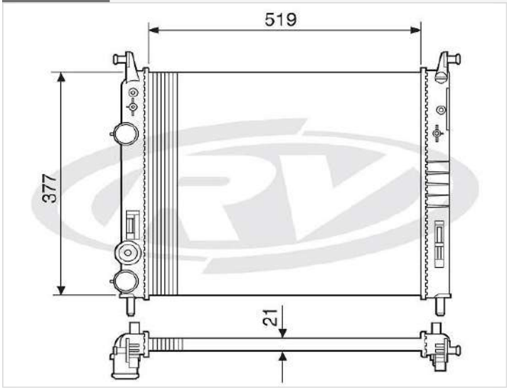
12540 FIAT
