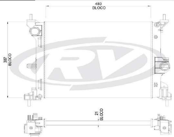
12544 FIAT
