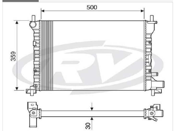
12583 FORD
