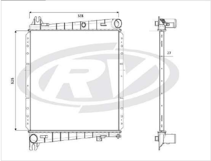
19275 FORD
