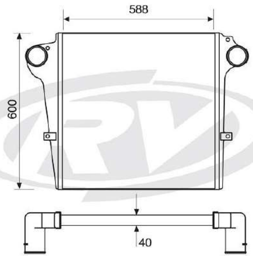
12273 FORD / VOLKSWAGEN
