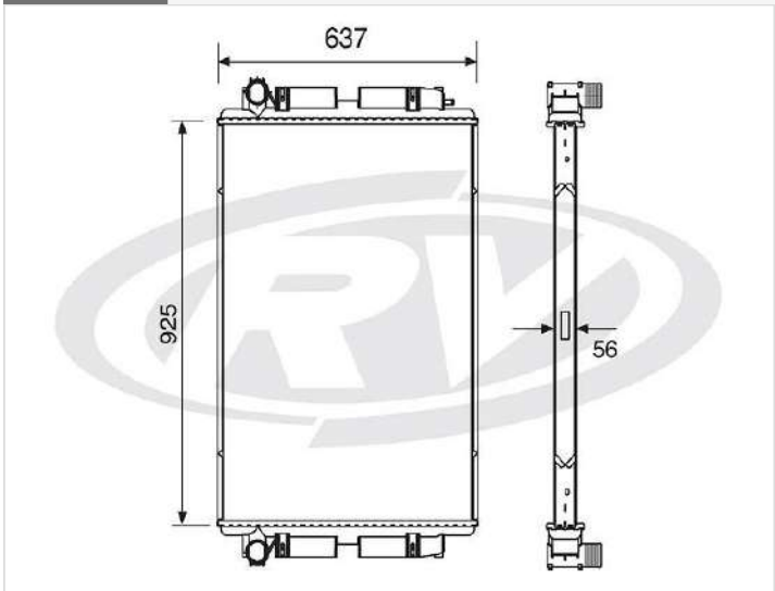
12003 MERCEDES - BENZ
