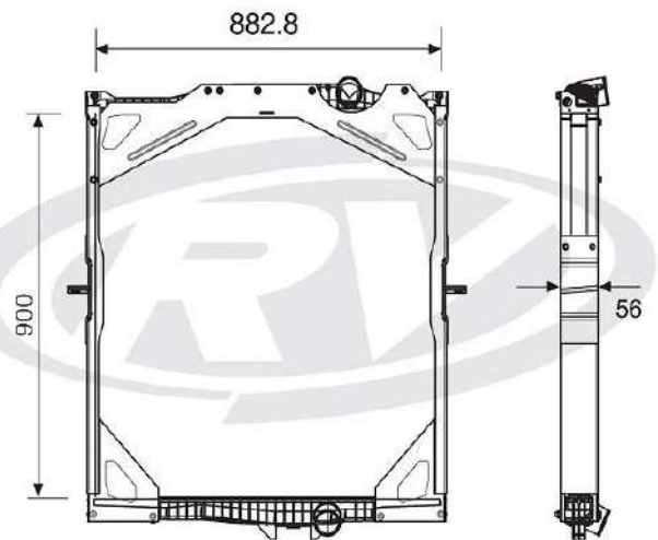
12061 VOLVO
