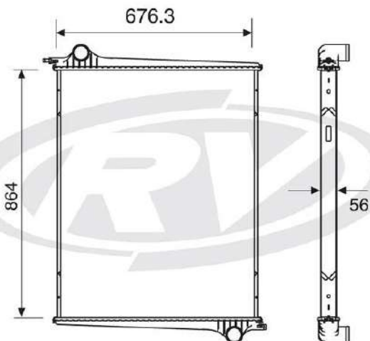
12045 SCANIA
