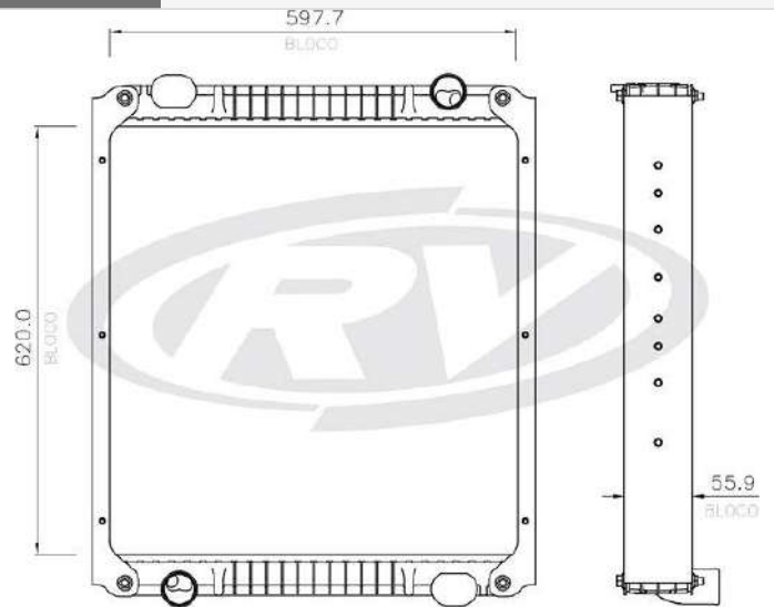
19903 AGRALE
