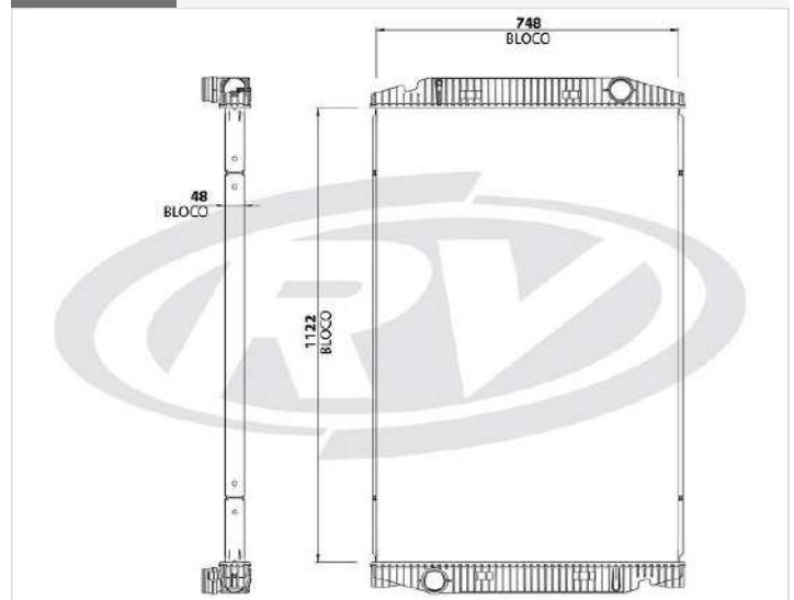
12084 IVECO
