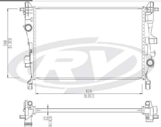
12548 FIAT
